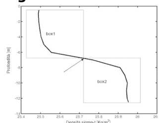
Figura 3.1 Relazione tra profondità e densità
